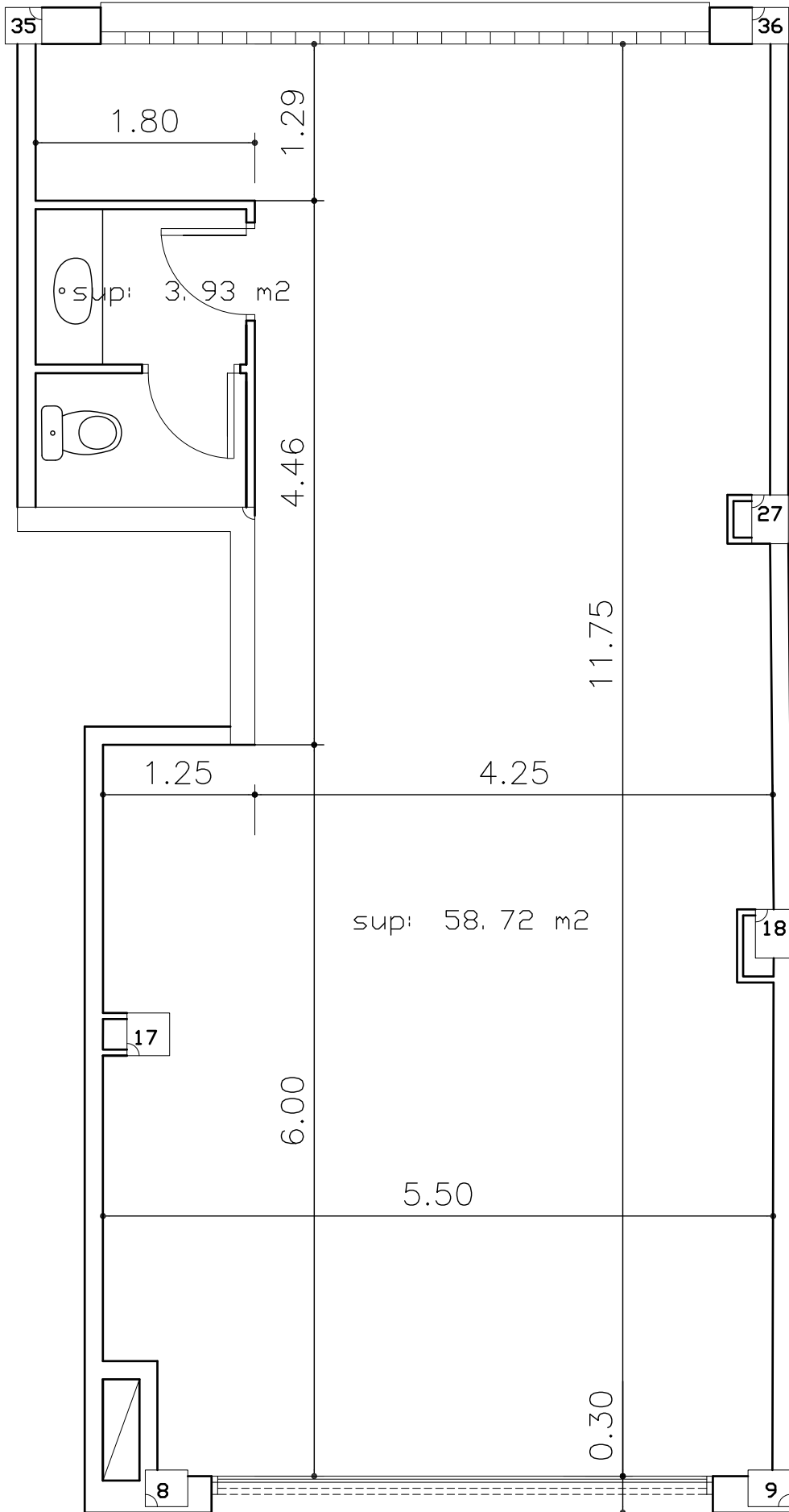
PLANTA LOCAL 5
