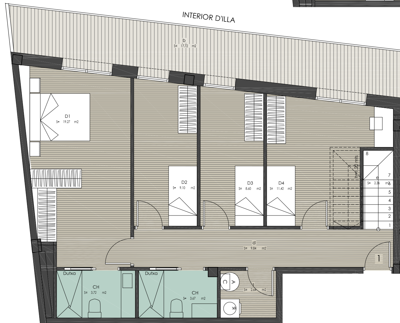
PLANTA SEGONA
