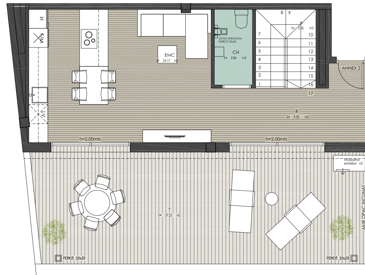
PLANTA SOTACOBERTA
